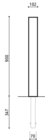
Piip 900 ajoestopollari - PP900
